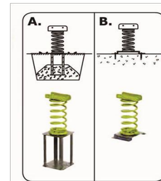
Sistema de anclaje según tipo de suelo
